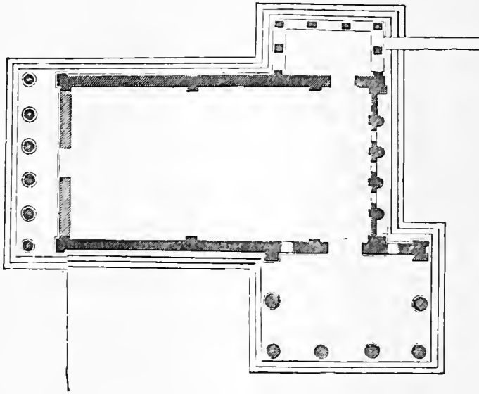
FIG. 73.—PLAN OF THE ERECHTHEIUM.
